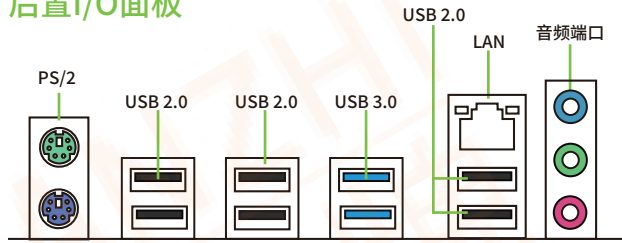
图1-2 整体后置I/O面板展示
